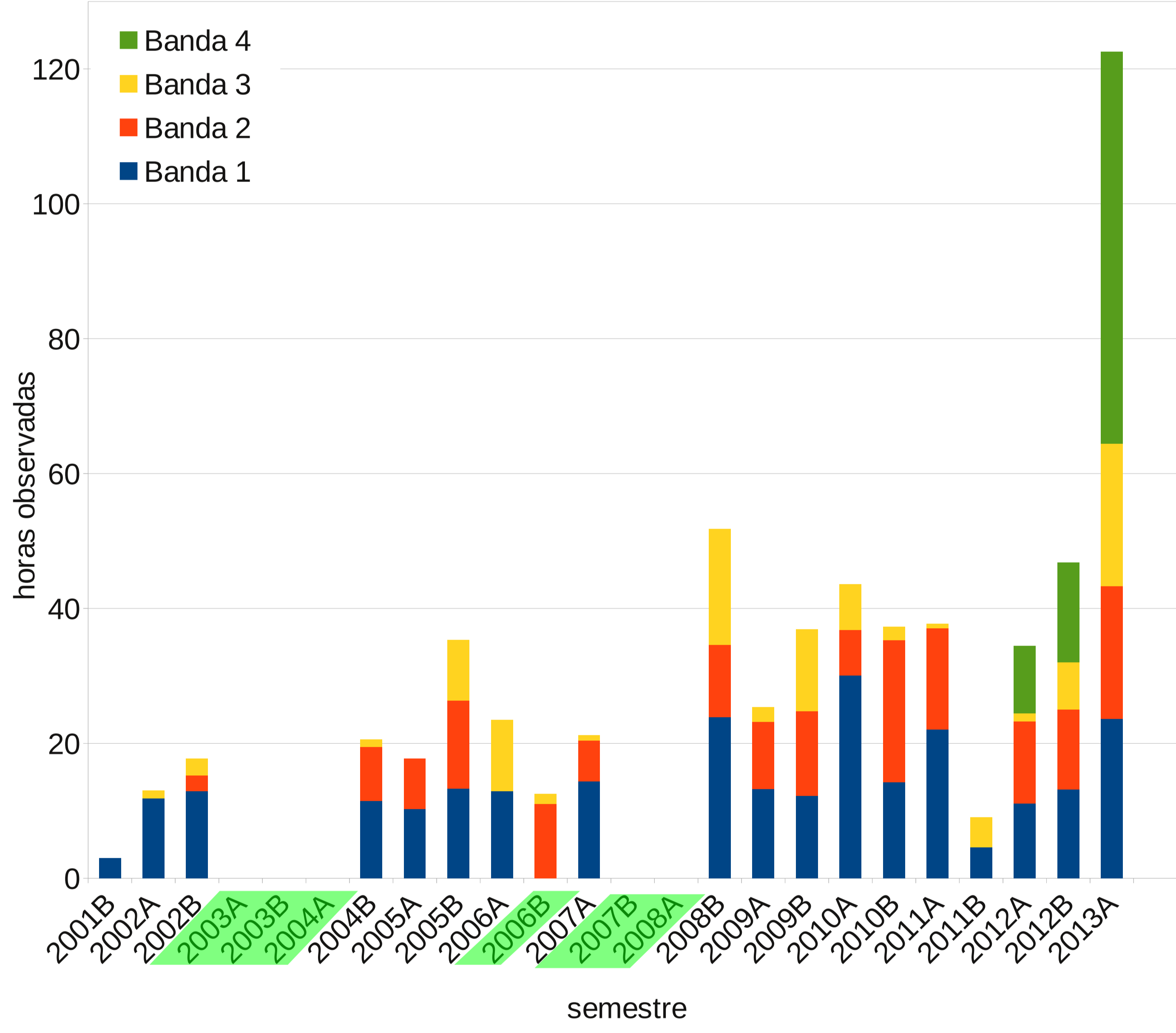
Evolución del tiempo observado (Gemini Norte + Sur) indicando bandas de condiciones de observación
