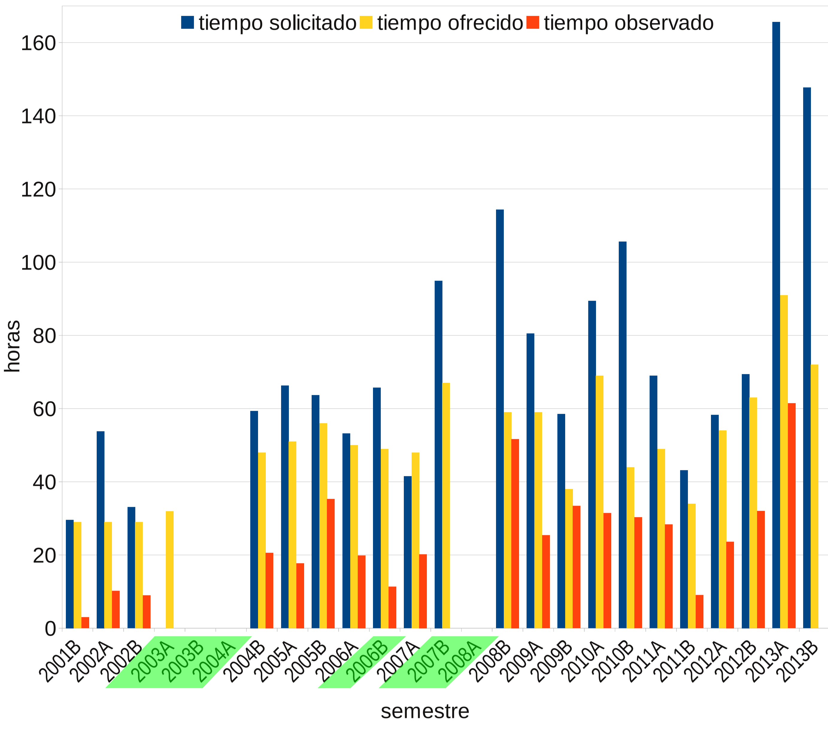
Evolución del tiempo observado (Gemini Norte + Sur) indicando bandas de condiciones de observación
